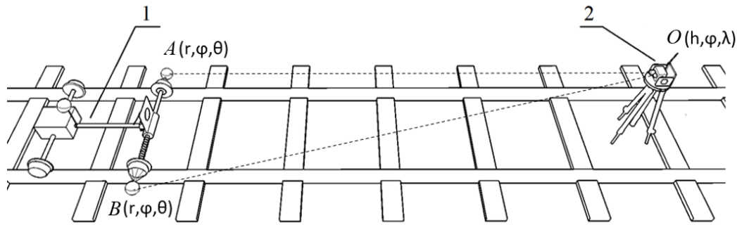
1 – путеизмерительная тележка; 2 – видеogramметрическое устройство; Рисунок 22 – Принципиальная схема размещения элементов ВСКЗ для контроля параметров геометрии рельсовой колеи
