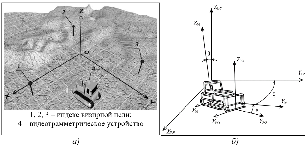
Рисунок 20 – Принципиальная схема размещения ВЦ на строительном участке (а), системы координат (б): видеограмметрического устройства ( X_{BV} Y_{BV} Z_{BV} ), строительной машины ( X_M Y_M Z_M ) и рабочего органа ( X_{PO} Y_{PO} Z_{PO} )
