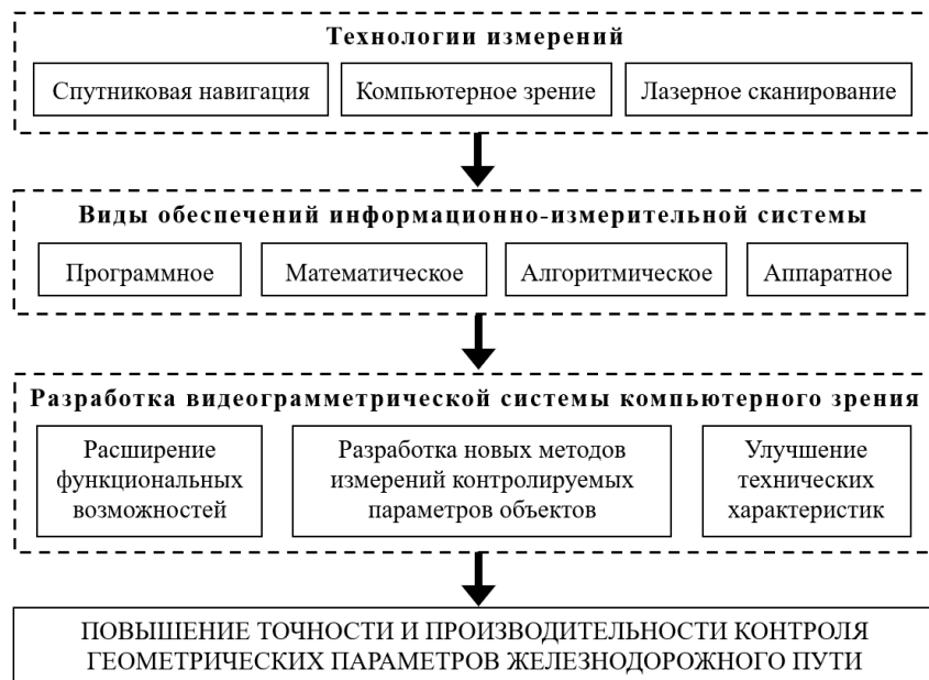
Рисунок 2 – Концепция разработки видеogramметрической системы на основе технологии компьютерного зрения
